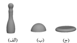
شکل 4 برخورد قطرات 2/3 میلی‌متری بر سطحی از جنس پارافیلیم M با سرعت برخورد 2m/s در زمان یکسان؛ (الف) آب، (ب) گلیسرین 50%، (ج) گلیسرین 80%
