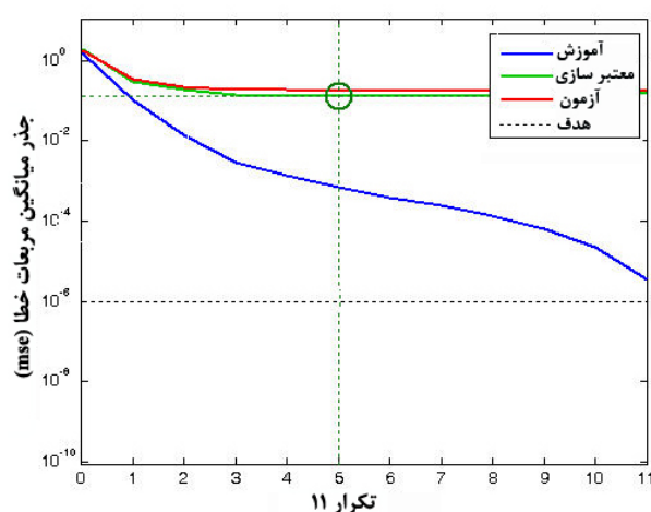
شکل ۱۰ روند تغییرات خطای MSE شبکه با استفاده از الگوریتم آموزشی لونبرگ-مارکوارت Trainlm
