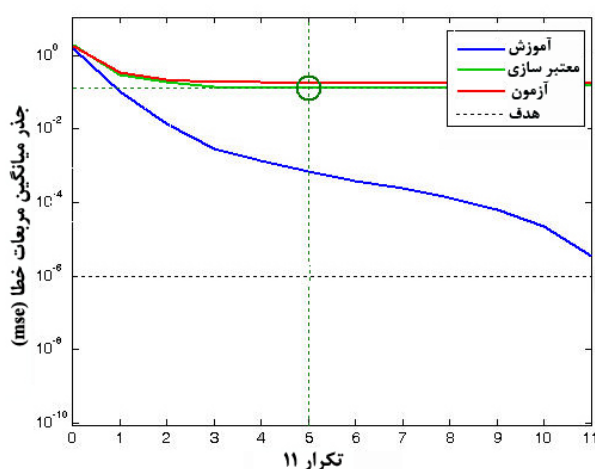
شکل ۱۰ روند تغییرات خطای MSE شبکه با استفاده از الگوریتم آموزش لونیگ-مارکوارت Trainlm
