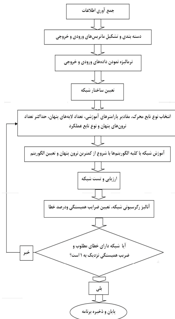
شکل ۳ مراحل ایجاد و انتخاب مدل پیش بینی عملکرد و آلاینده
