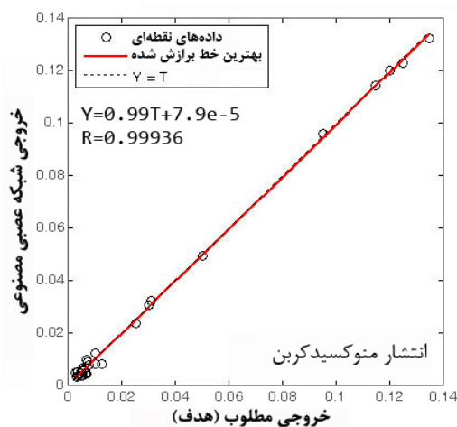
شکل ۱۴ آنالیز رگرسونی میان خروجی شبکه و خروجی مطلوب برای پیش‌بینی انتشار آلاینده‌های مونوکسید کربن
