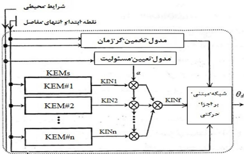
شکل 3 نمای کلی الگوریتم MHMP [22]
