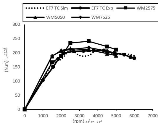
شکل ۹) منحنی گشتاور در حالات مختلف
