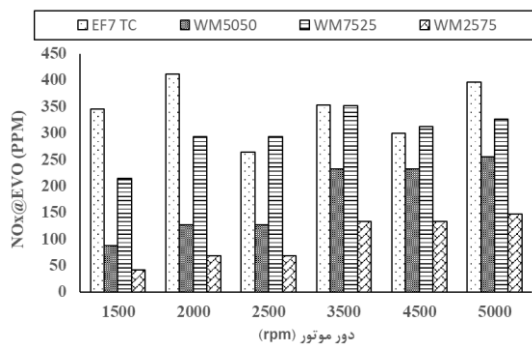
شکل ۶) مقایسه انتشار آلاینده اکسیدهای نیتروژن خارج شده از آگروز در دور موتورهای مختلف [14]
