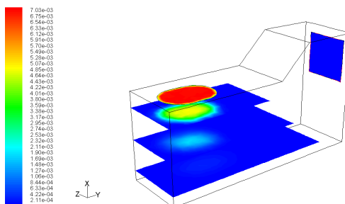
شکل ۹ کسر جرمی مونوکسیدکربن ( CO ) در داخل محفظه ته‌نشین کننده ذرات
