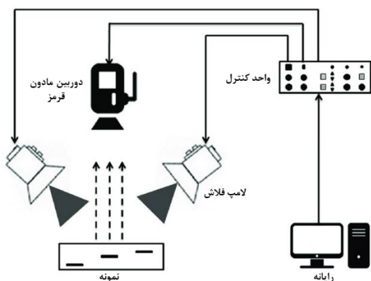
شکل ۱) تجهیزات تصویربرداری
