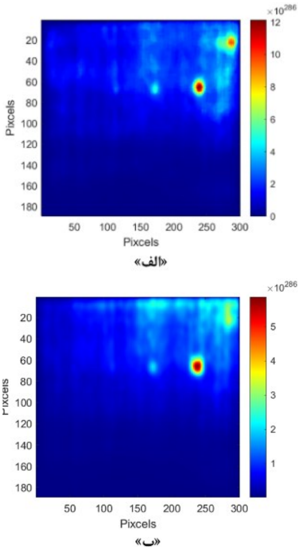
شکل ۴ مقایسه فیلتر میانه و گاوسین، «الف» اضافه شدن فیلتر میانه با اندازه همسایگی ۹ در ۹ روی تصویر حاصل از فیلتر حذف تصویر زمینه با درجه فیلتر ۲۰۰، «ب» اضافه شدن فیلتر گاوسین با سیگما سه روی تصویر حاصل از فیلتر حذف تصویر زمینه با درجه فیلتر ۲۰۰
