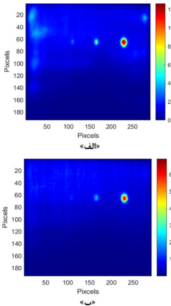
شکل ۶ مقایسه فیلتر میانه و گاوسین، «الف» اضافه شدن فیلتر میانه با اندازه همسایگی ۷ در ۷ روی تصویر حاصل از فیلتر حذف تصویر زمینه با درجه فیلتر ۱۰۰، «ب» اضافه شدن فیلتر گاوسین با سیگما یک روی تصویر حاصل از فیلتر حذف تصویر زمینه با درجه فیلتر ۱۰۰
