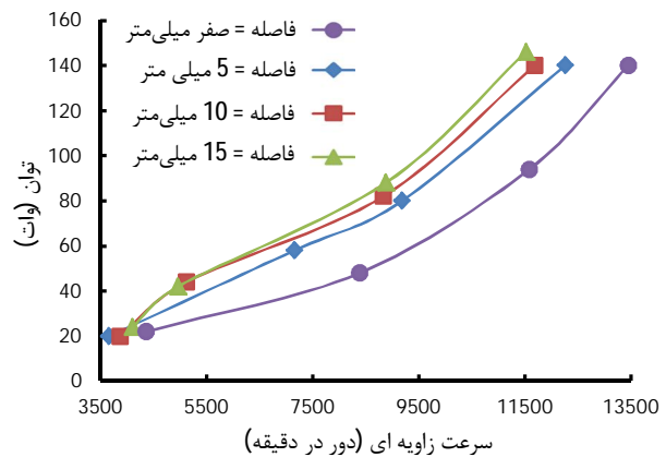
شکل 9 تغییرات توان ورودی بر حسب سرعت دورانی، در فاصله‌های مختلف جاذب از سطح
