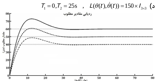
شکل 13 ردیابی مقادیر مطلوب - ضریب مشاهده‌گر اغتشاش بزرگ
