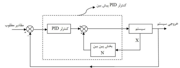
شکل 2 دیاگرام بلوکی کنترلر PID پیش بین
