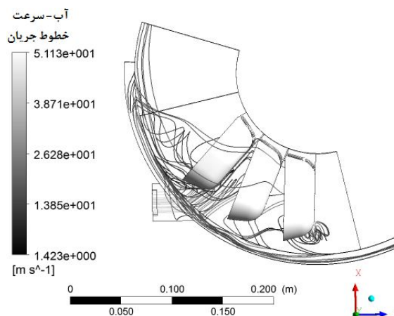
شکل ۱۶ خطوط جریان برای فاصله افقی ۱۶۵ میلی‌متر
