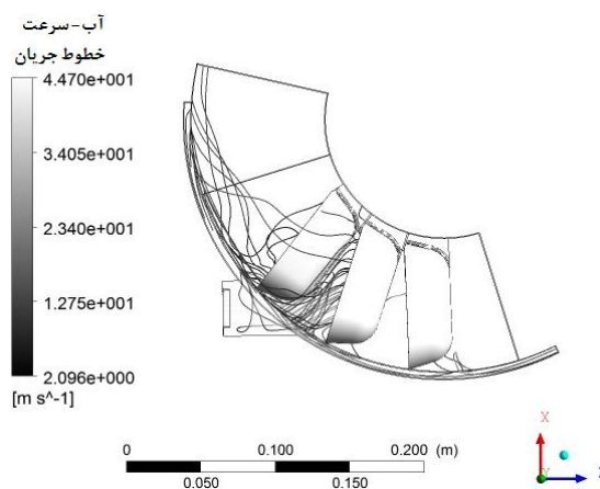
شکل ۱۵ خطوط جریان برای فاصله افقی ۱۵۰ میلی‌متر
