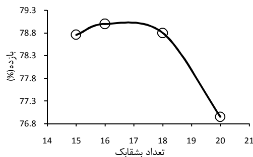
شکل ۱۷ تاثیر تعداد بشقابک با اندازه و قطر گام ثابت بر بازده
