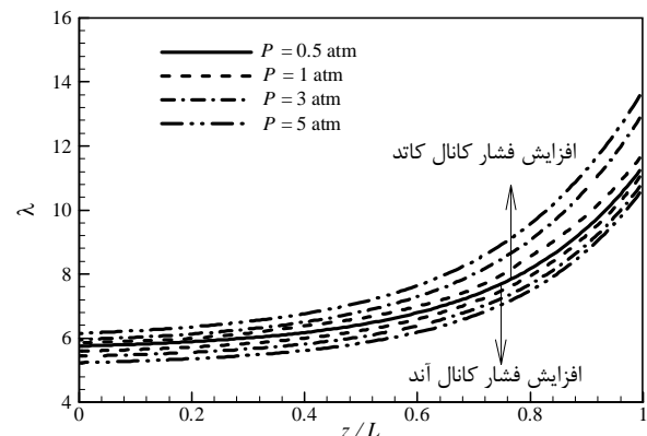
شکل 15 منحنی تغییرات محتوای آب غشاء به ازای فشار گاز ورودی به کاتد و آند متفاوت در چگالی جریان 1 A/cm^2
