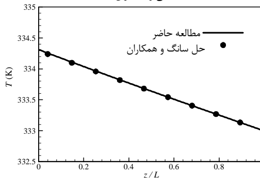
شکل 3 مقایسه منحنی توزیع درجه حرارت در کاند پیل سوختی حاضر
