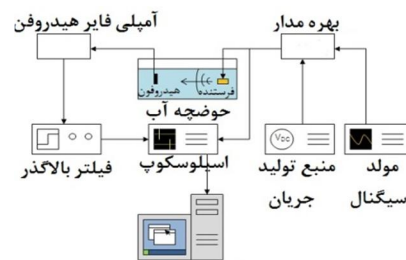
شکل 15 سیستم ارزیابی عملکرد آکوستیکی یک ترانسدیوسر
