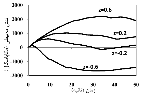
شکل ۱۳ نمودار تغییرات تنش هوپ بر حسب زمان
