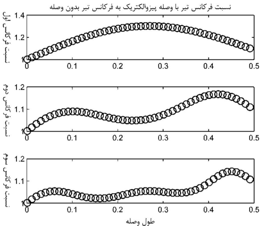
شکل 13 نحوه اثرگذاری وصله پیزوالکتریک بر فرکانس تیر در طول‌های مختلف
