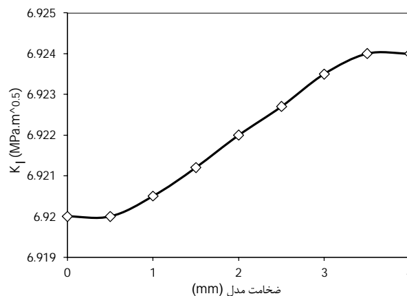
شکل 6 تغییرات ضریب شدت تنش مود یک در راستای ضخامت ورق با شعاع انحنای r = 1 m
