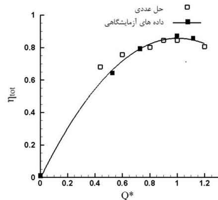
شکل 7 مقایسه منحنی مشخصه راندمان کل - دبی برای حل عددی و داده‌های آزمایشگاهی
