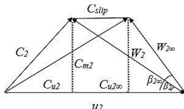
شکل 2 مقایسه کلی بین مثلث‌های سرعت واقعی و تئوری در خروجی چرخ [16]
