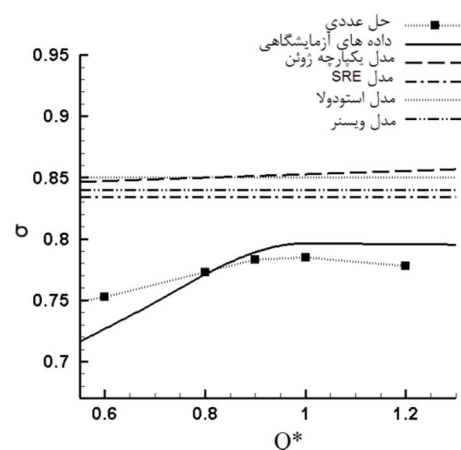
شکل 11 بررسی تغییرات ضریب لغزش با دبی توسط مدل‌های مختلف
