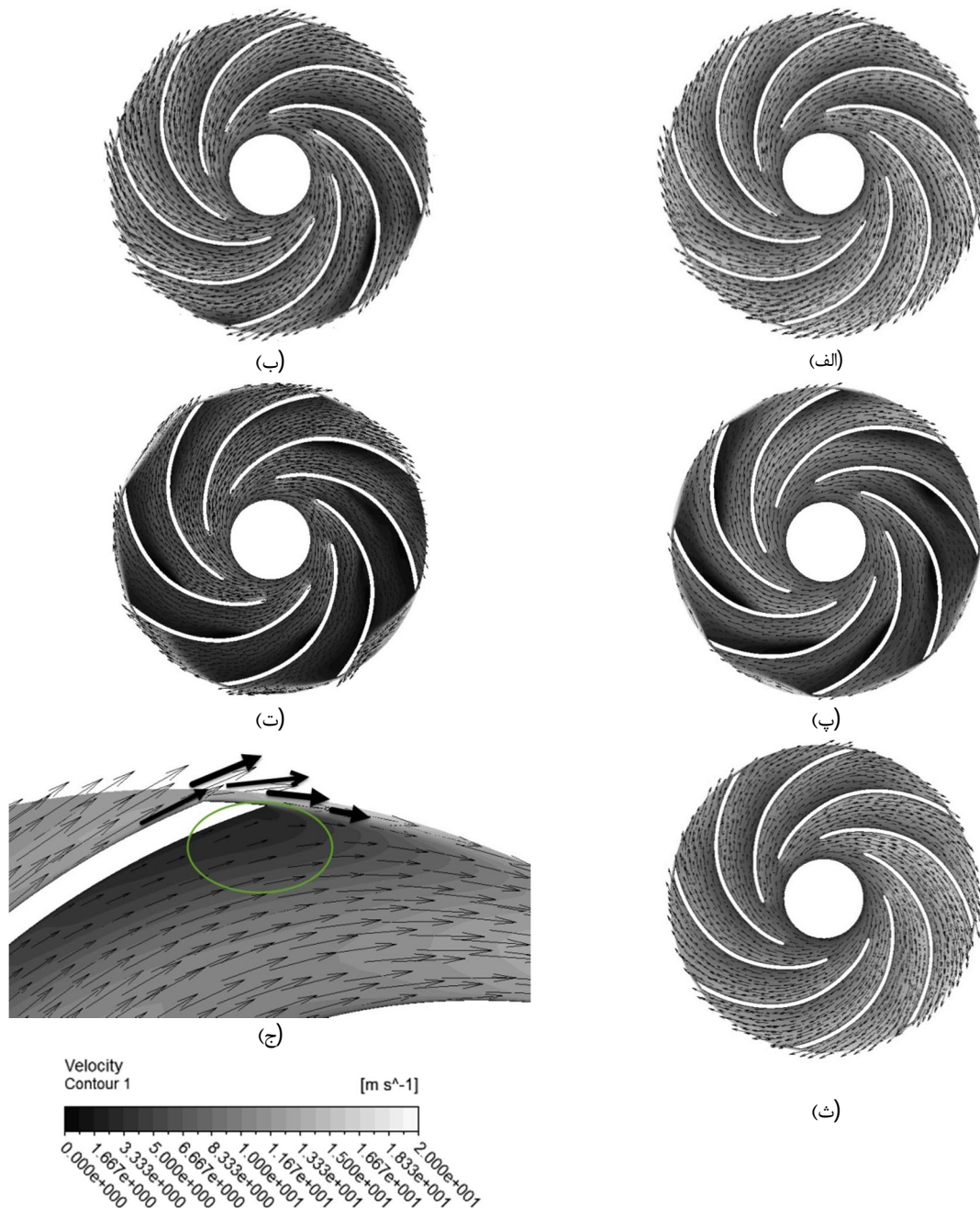
شکل 10 بردارها و کانتورهای سرعت نسبی برای دبی‌های مختلف (الف) Q^*=1 (ب) Q^*=0.8 (پ) Q^*=0.6 (ت) Q^*=0.45 (ث) Q^*=1.2 (ج) جزئیات در خروجی پره و اثر واماندگی جریان بر مسیر حرکت ذرات سیال و ضریب لغزش
