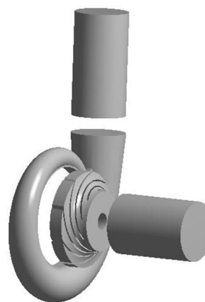
شکل 1 اجزای پمپ شبیه‌سازی شده
